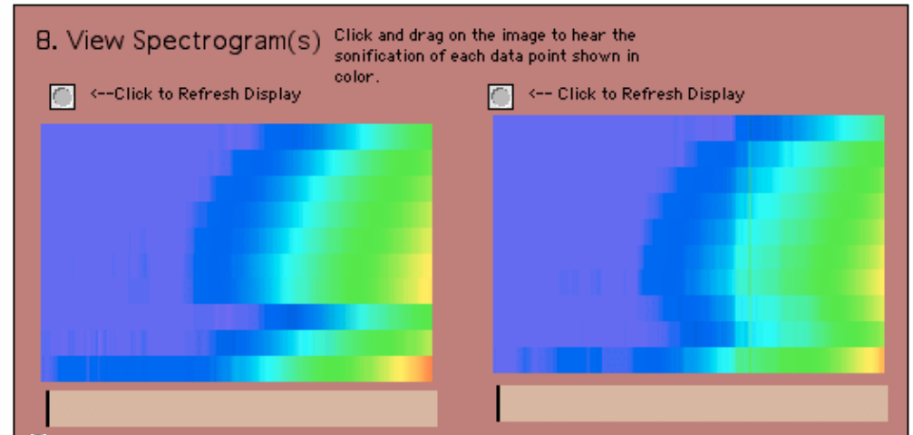
LET CME, Dec. 6 + 40 hrs
